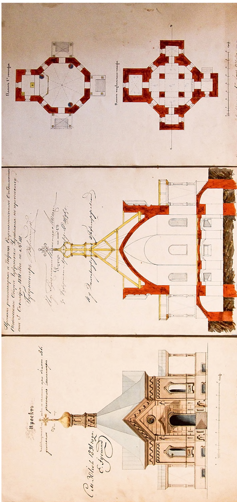
Ил. 1. Проект Кладбищенской церкви (НА ТИАМЗ № ТМ-11794/10)
