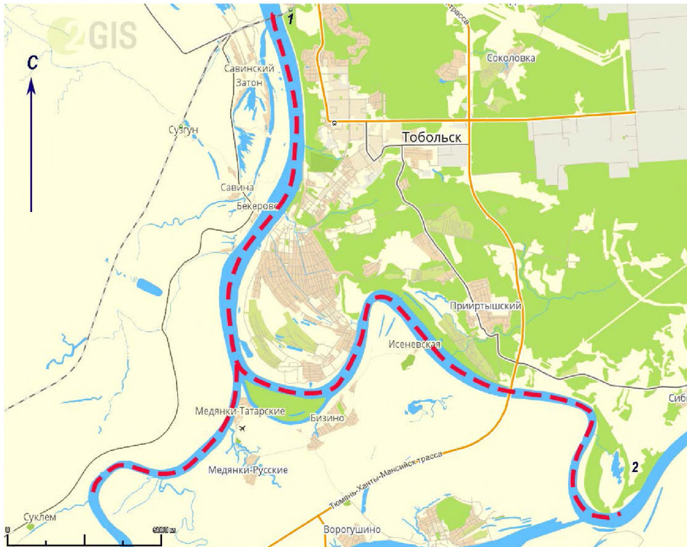
Рисунок 1 – Реконструкция маршрута путешествий Романовых по рекам Иртыш и Тобол и мест посещения в августе 1917 г. Примечание: 1-2 – памятники археологии (1- Сузгунская гора (Сузгун I-II), 2 – Саускановская гора (Ханское кладбище))
